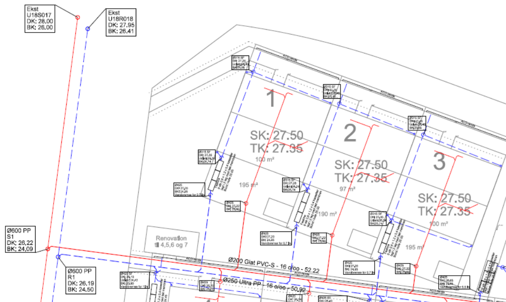
Figur 2: Udklip fra kloaktegnning. Herregårdsparken 6 er placeret på felt 3. Faskine til forsinkelse af regnvand etableres i det sydvestlige hjørne af matriklen. Vandbremse etableres før tilslutning til regnvandsledning i Husoddevej.
