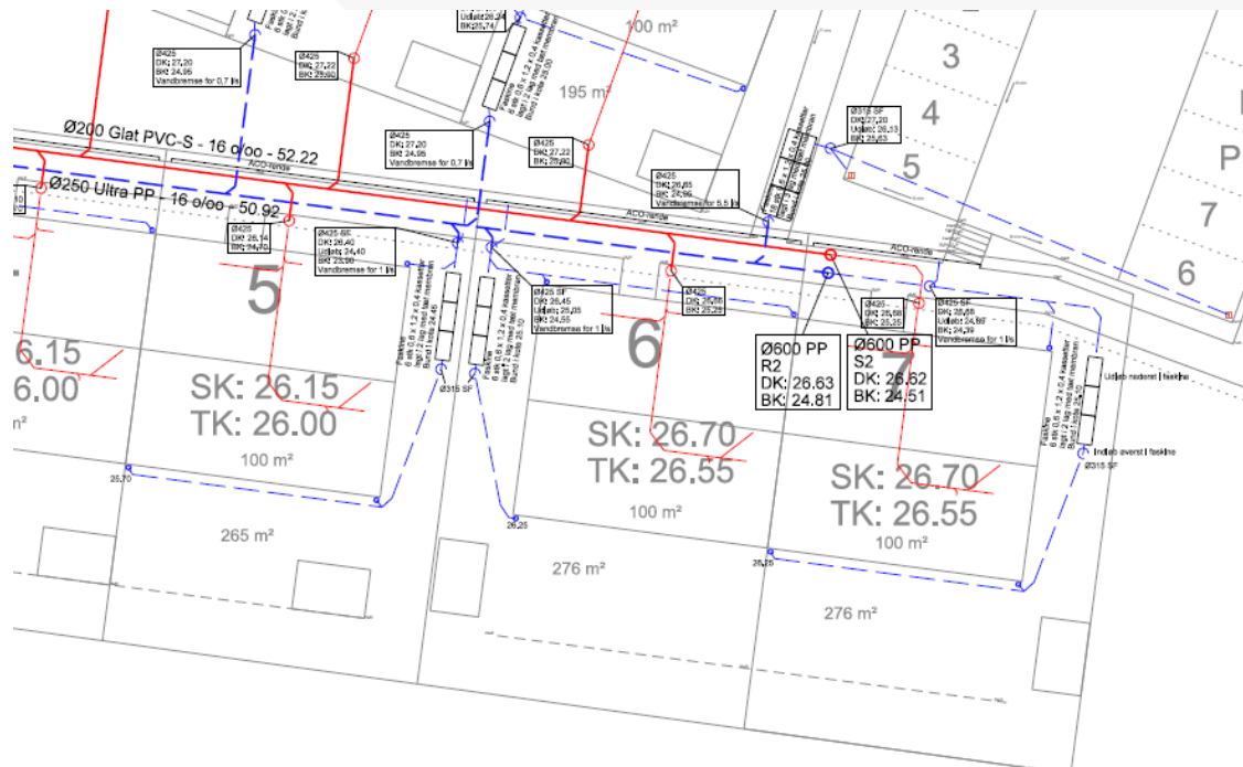
Figur 2: Udklip fra kloaktegning. Herregårdsparken 14 er placeret på felt 7. Faskine til forsinkelse af regnvand etableres på østsiden af byggeriet. Vandbremse etableres før tilslutning til regnvandsledning i Husoddevej.
