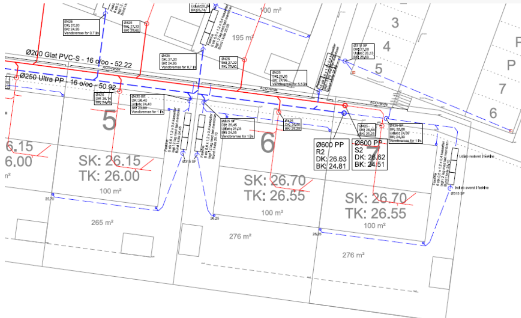
Figur 2: Udklip fra kloaktegning. Herregårdsparken 12 er placeret på felt 6. Faskine til forsinkelse af regnvand etableres på vestsiden af byggeriet. Vandbremse etableres før tilslutning til regnvandsledning i Husoddevej.
