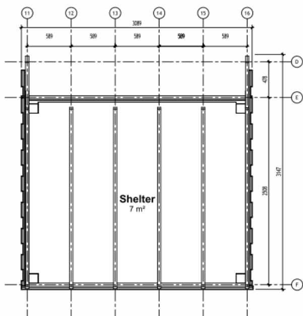
Plan, Shelter 1 : 25
