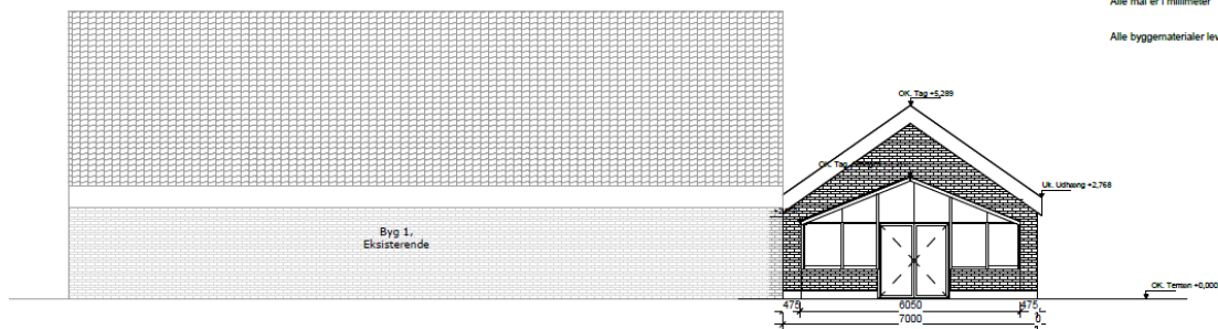
Syd 1:100
