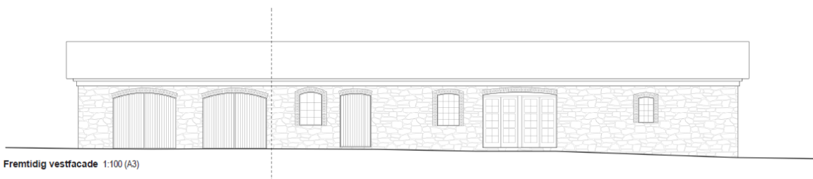
Eksisterende vestfacade 1:100 (A3)
