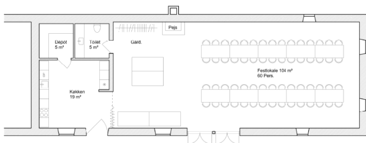
Fremtidig plan 1:100 (A3)
