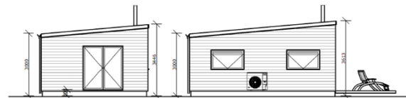
● Facade mod Øst 1 : 100
