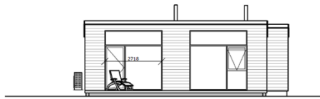
● Facade mod syd 1 : 100
