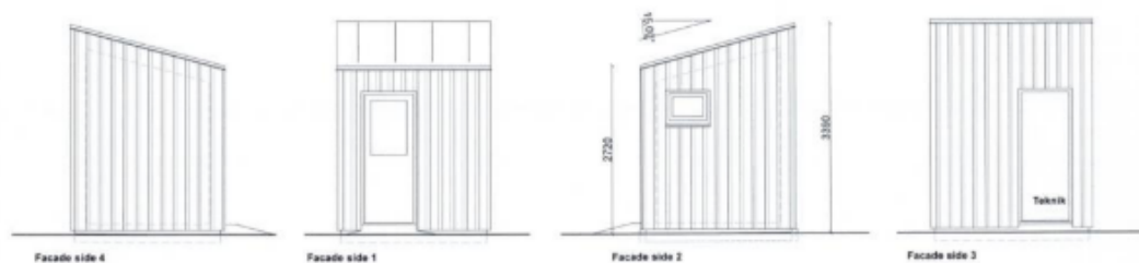
Fig. 4. Tilsendt fra ansøger. På figuren ses en illustration af facaderne på de mobile badeværelser.
