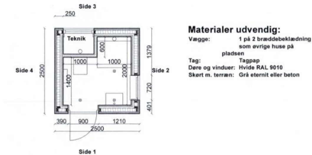
Fig. 3. Tilsendt fra ansøger. På figuren ses en plantegning over de ansøgte mobile badeværelser, der er indrettet med bruser, toilet, og håndvask. Der er derudover et teknikrum.
