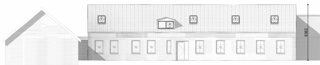
FACADE MOD SYD 1 : 100
